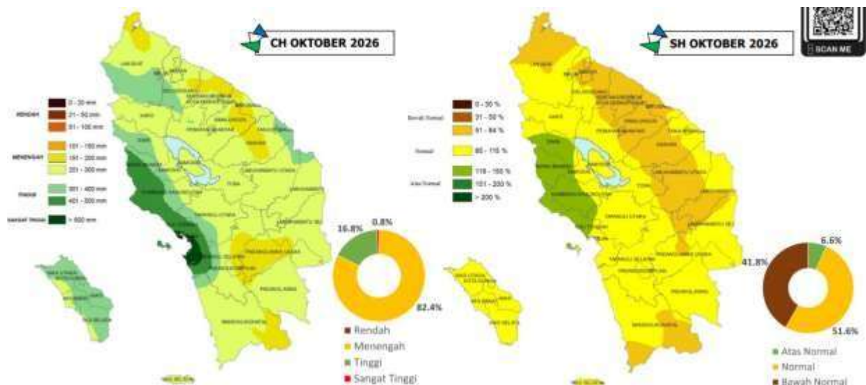
Gambar 2.5.3 Prakiraan Curah Hujan dan Sifat Hujan Oktober 2026
