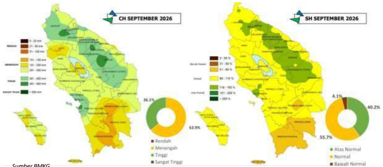
Gambar 2.5.2 Prakiraan Curah Hujan dan Sifat Hujan September 2026
