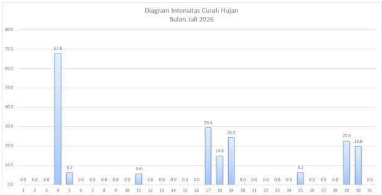
Gambar 2.1.3.1 Intensitas Curah Hujan Bulan Juli 2026
