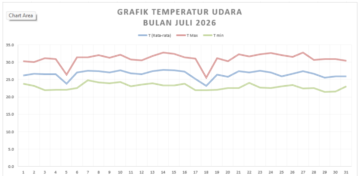
Gambar 2.1.1.1 Grafik Suhu Udara Bulan Juli 2026
