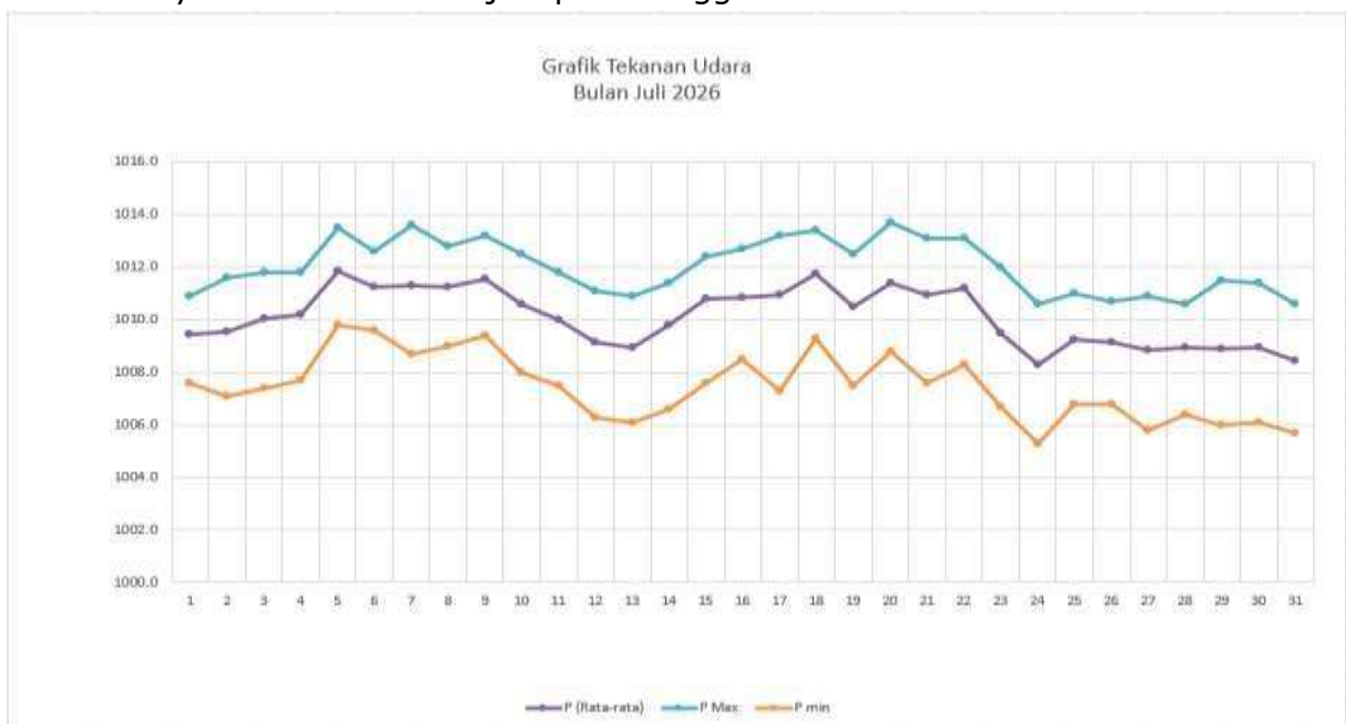
Gambar 2.1.4.1 Grafik Tekanan Udara Bulan Juli 2026
