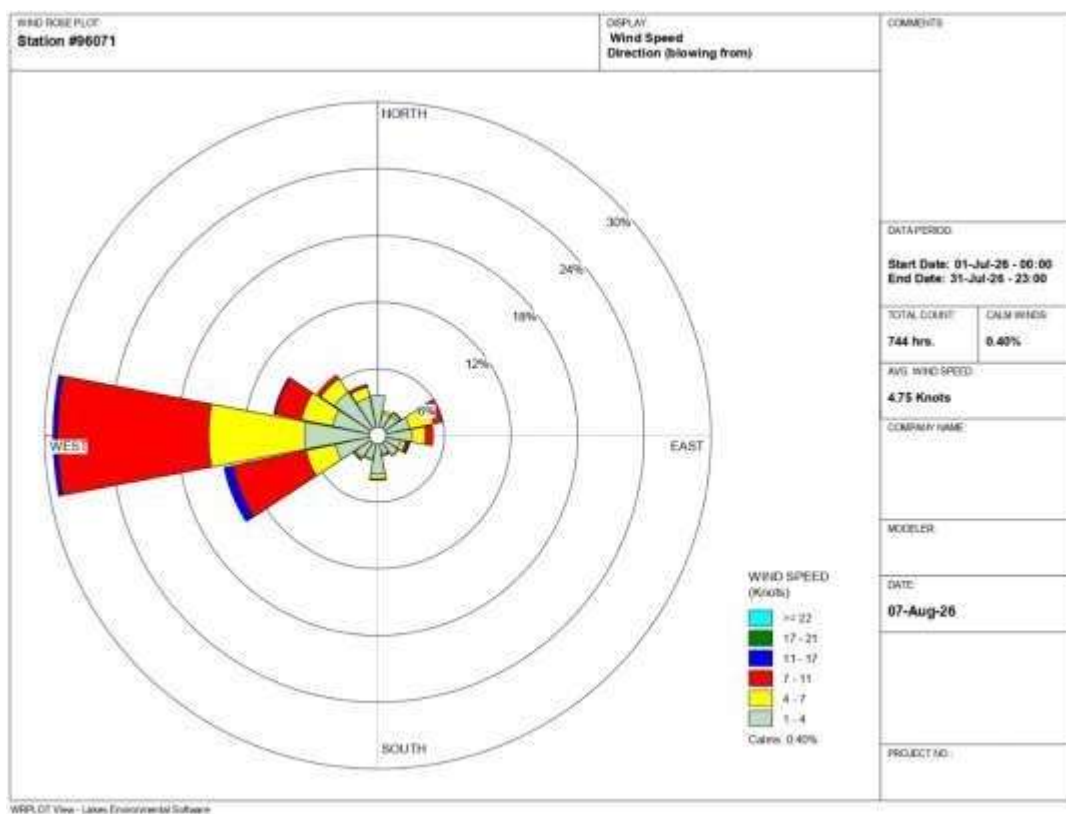
Gambar 2.1.6.1 Grafik Angin Bulan Juli 2026
