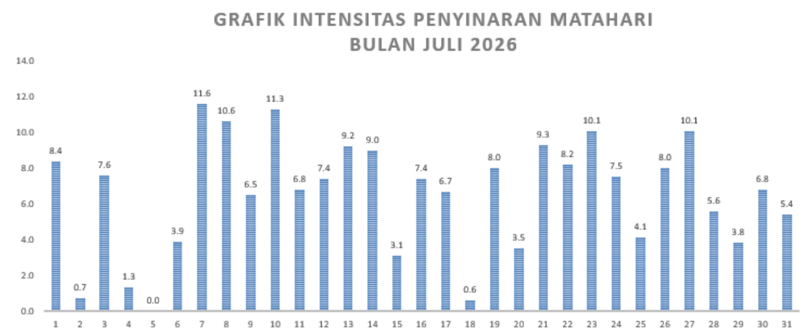
Gambar 2.1.2.1 Grafik Durasi Penyinaran Matahari Bulan Juli 2026
