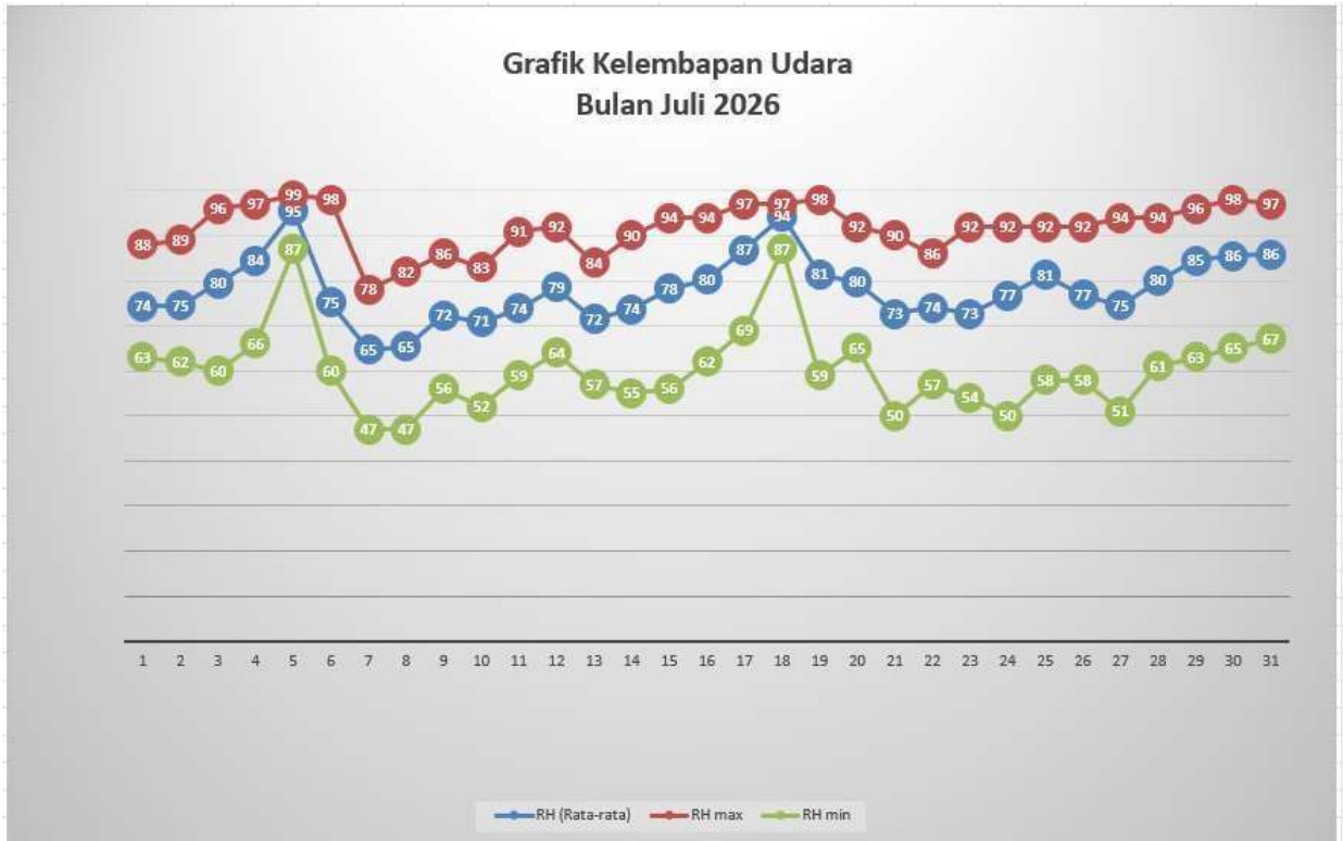
Gambar 2.1.5.1 Grafik Kelembaban Udara Bulan Juli 2026
